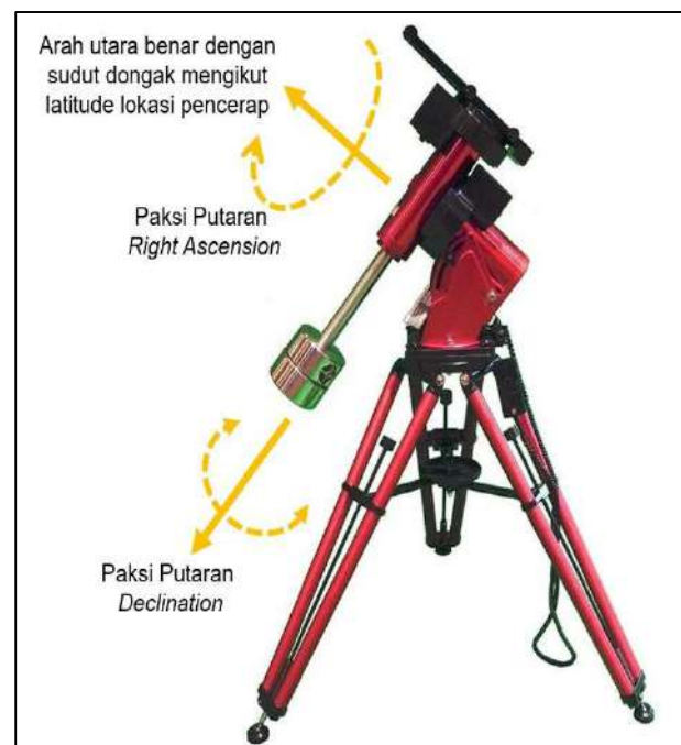
Imej 4: Pelekap/Pejejak Jenis Equatorial
